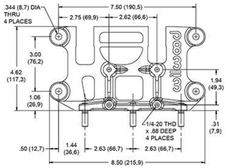
VIEW A-A
